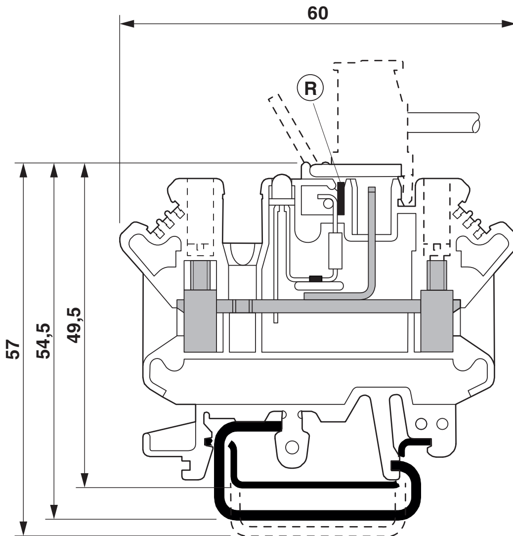
Dessin coté
