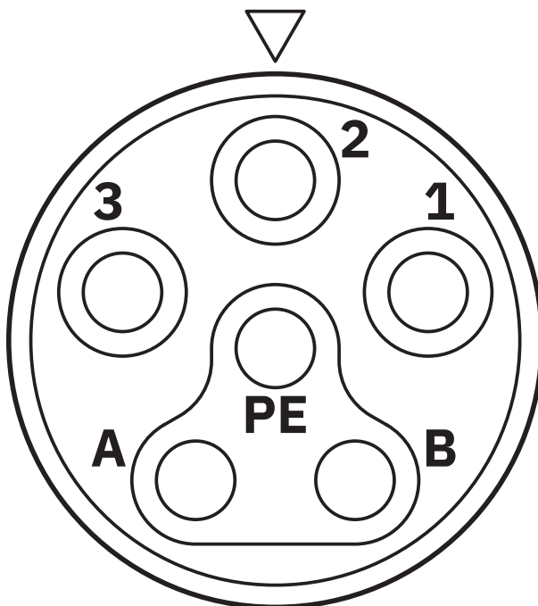
Esquema de polos de conector hembra M15, 6 polos, vista: lado de hembras
