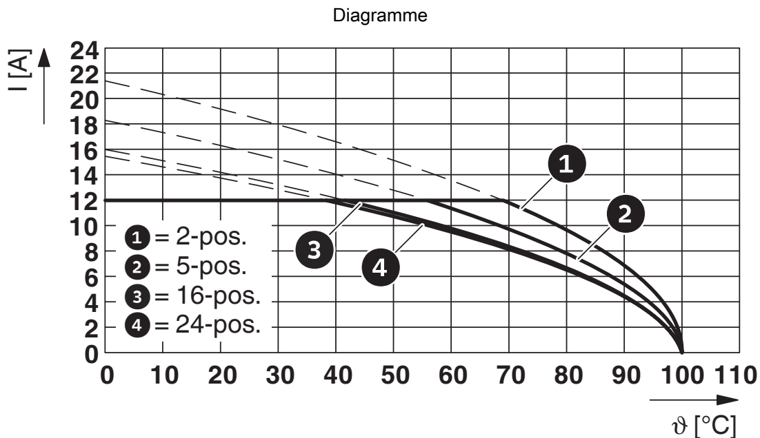
Type : SMSTB 2,5/...-STF avec MSTB 2,5/...-GF-5,08
