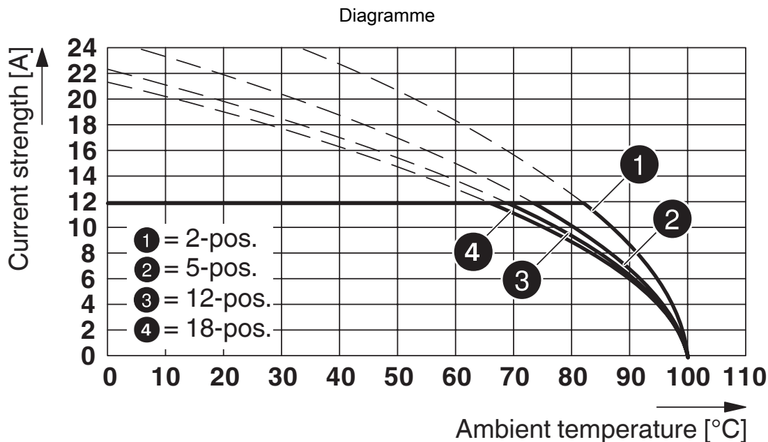
Type : FKCT 2,5/...-STF avec MSTB 2,5/...-GF-5,08
