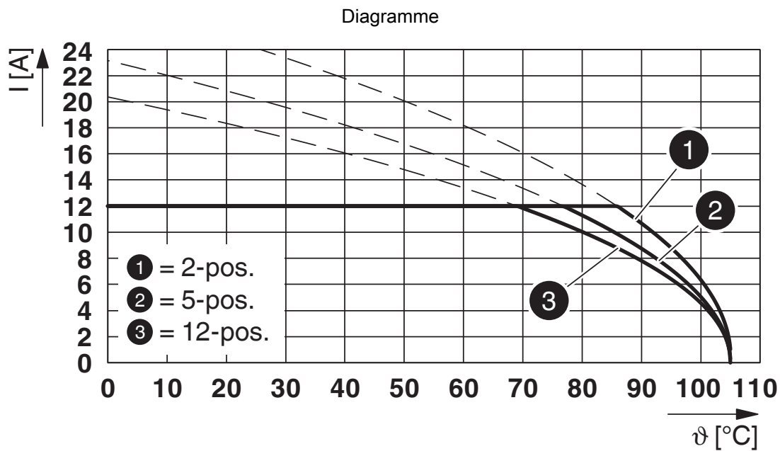
Type : FKCVR 2,5/...-STF-5,08 avec MSTB 2,5/...-GF-5,08
