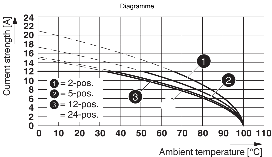
Type : MVSTBR 2,5/...-STF-5,08 avec MSTB 2,5/...-GF-5,08
