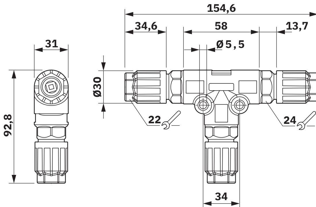
Maßzeichnung
