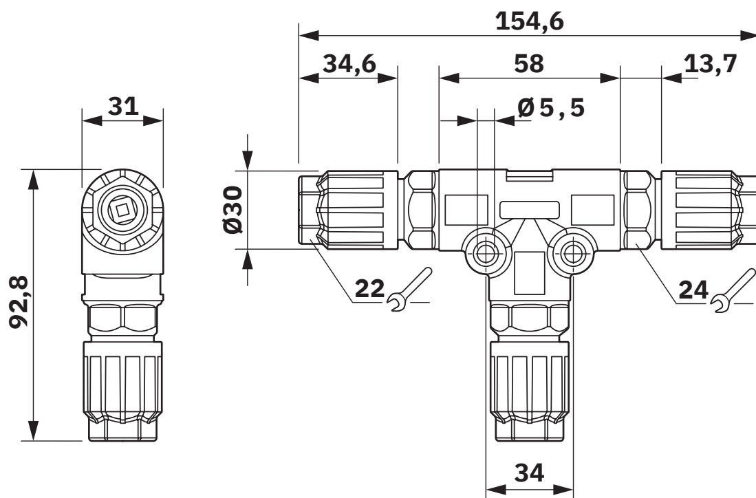
Dessin coté
