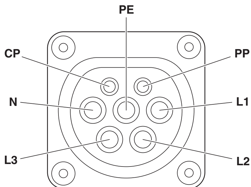
Anschlusszeichnung
