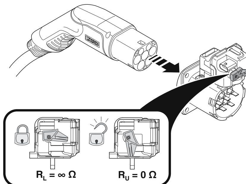
Positionen des Notentriegelungshebels des Verriegelungsaktors
