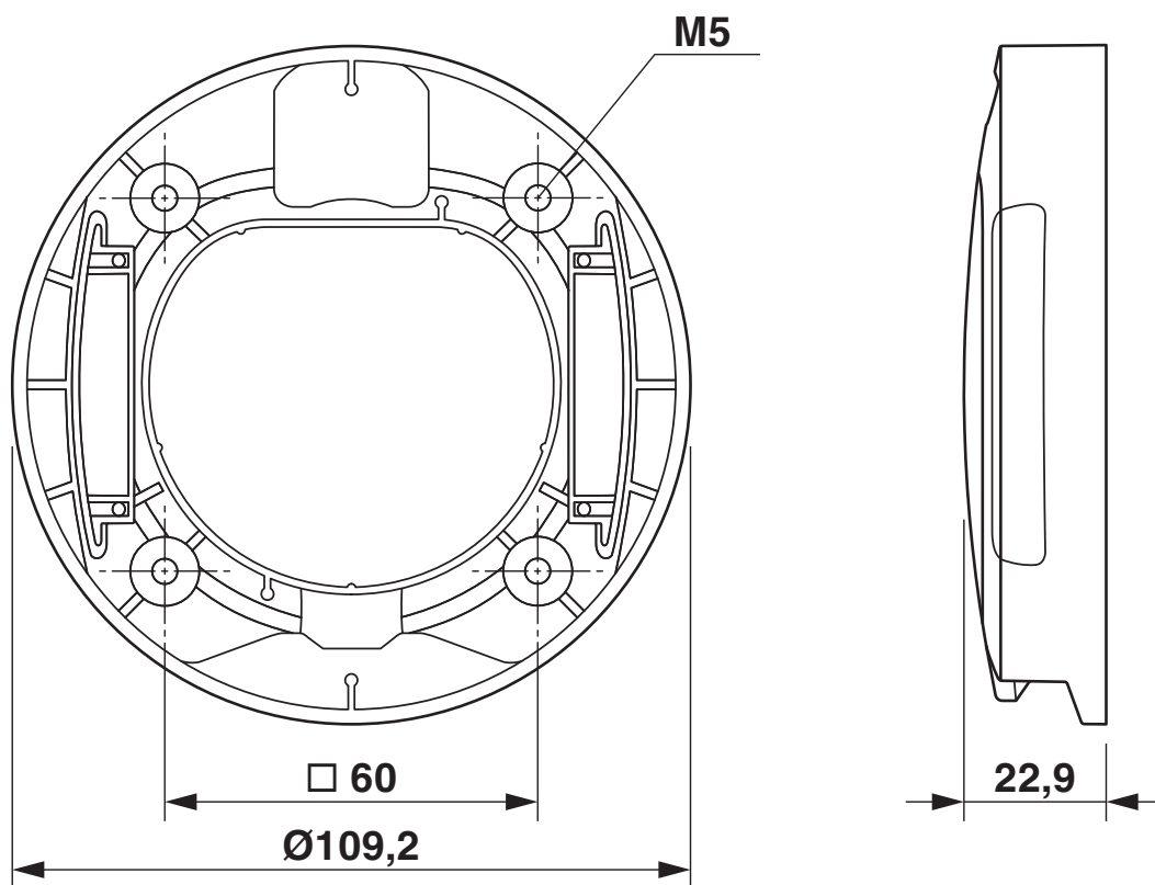
Dessin coté
