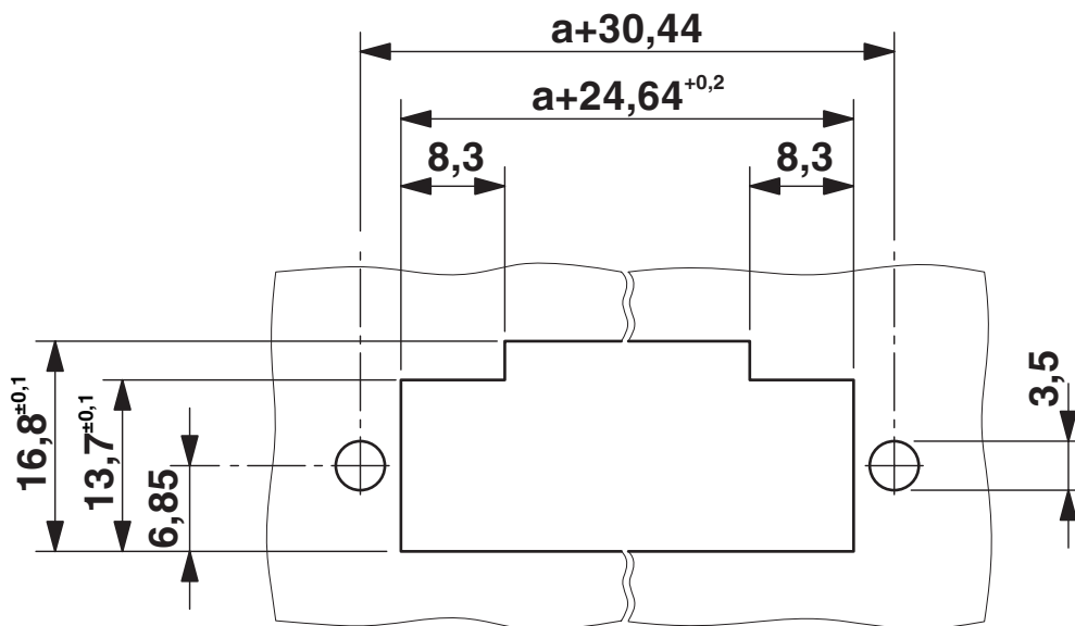
Maßzeichnung
