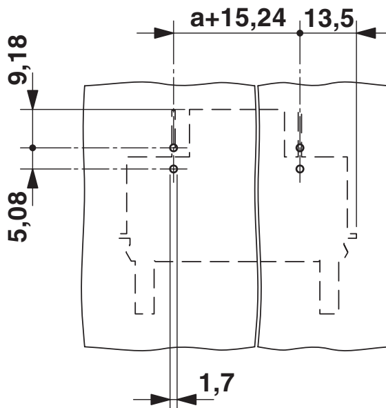
Bohrplan/Lötpadgeometrie
