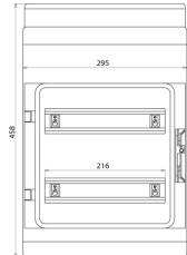
Dimensiones de IGA 24 IP54
