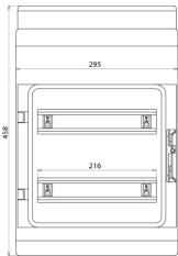
Dimensioni IGA 24 IP54
