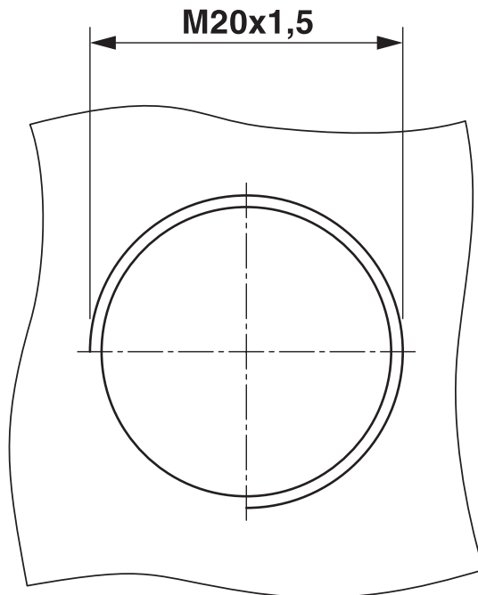
Dessin coté
