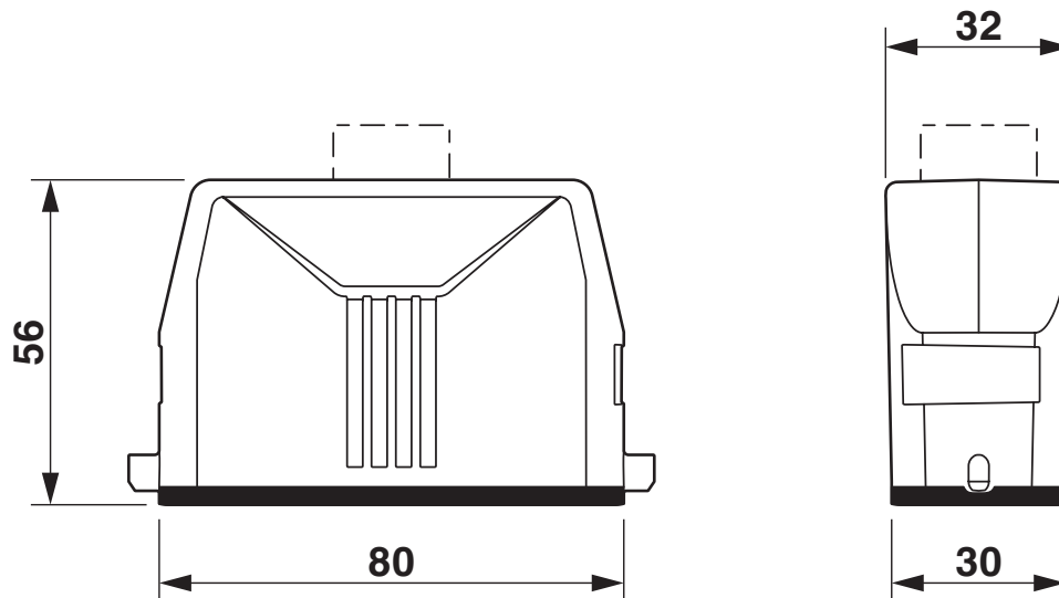
Maßzeichnung
