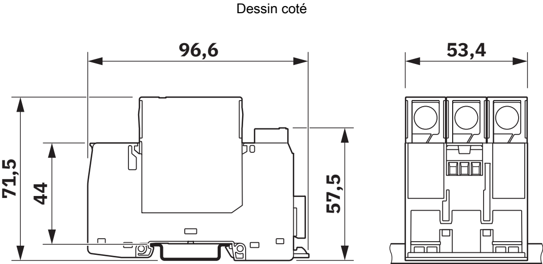
Dessin schématique
