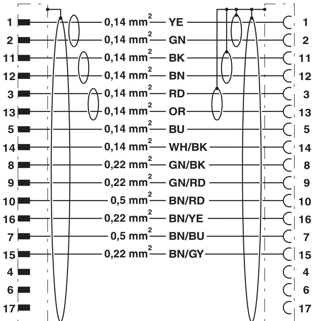
Schaltplan
