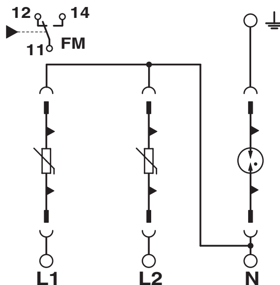
Diagrama eléctrico
