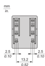
Stecker-Seitenansicht
