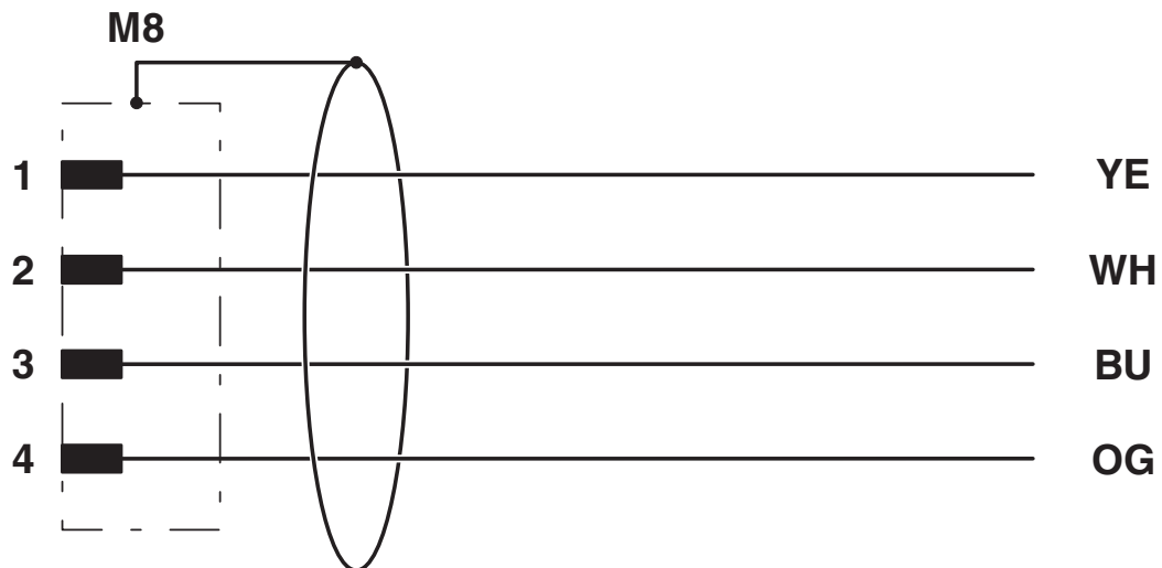
Diagrama eléctrico
