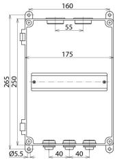
Dimensiones de IIGA 7 IP54
