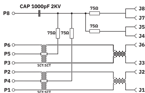
Schaltplan
