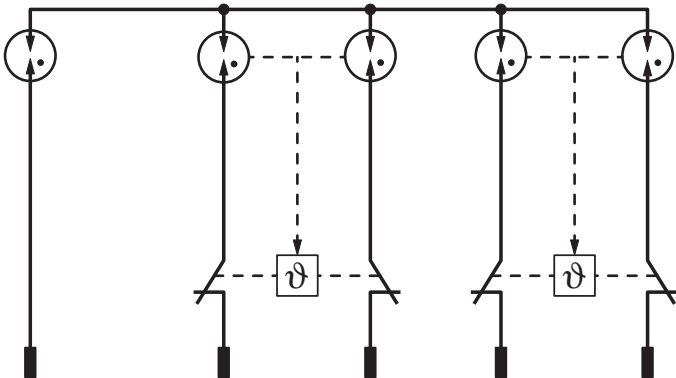
Schéma de connexion
