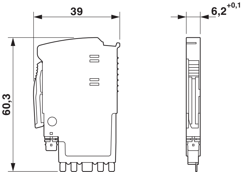
Dessin coté
