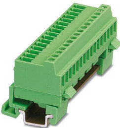
La figura muestra una variante de 16 polos
