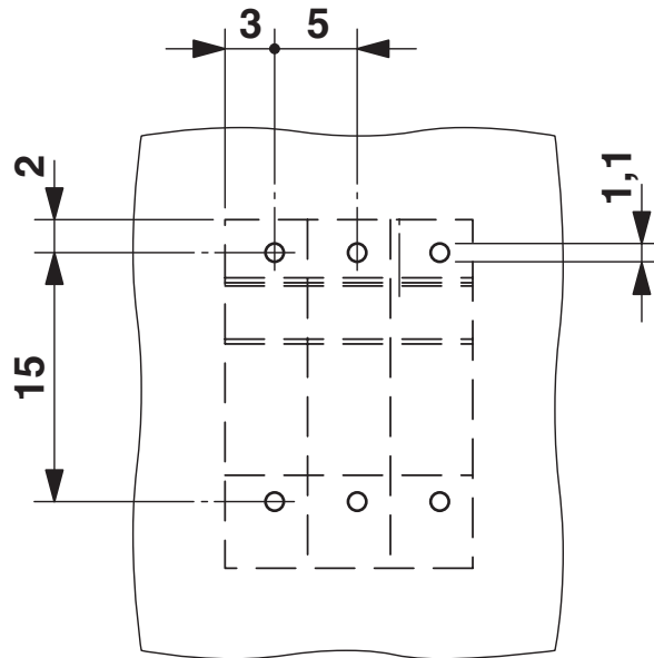
Bohrplan/Lötpadgeometrie
