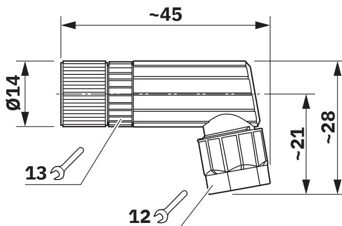
Esquema de dimensiones
