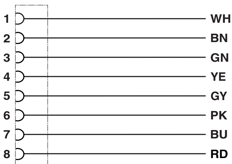
Diagrama eléctrico
