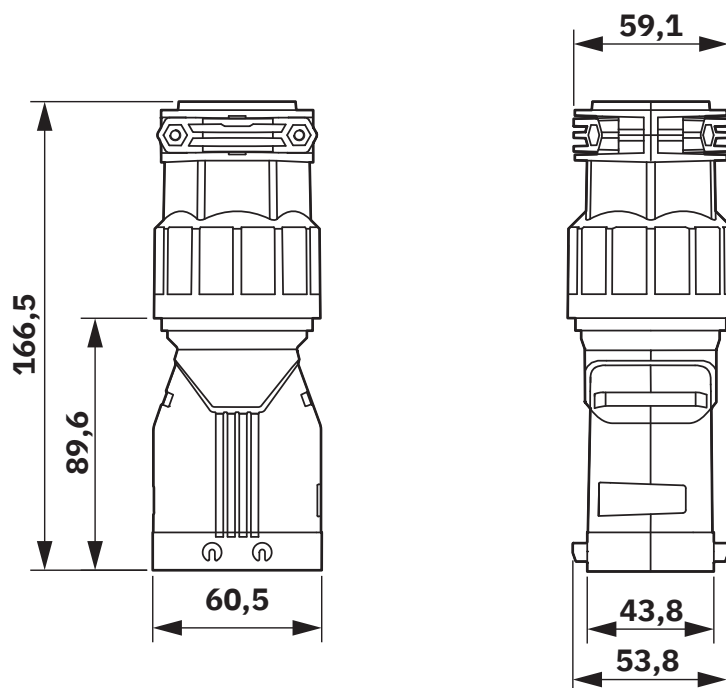
Dessin coté
