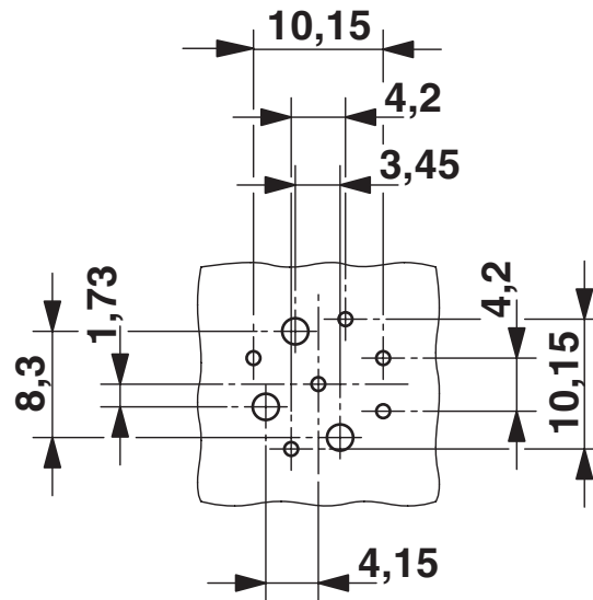
Bohrplan/Lötpadgeometrie
