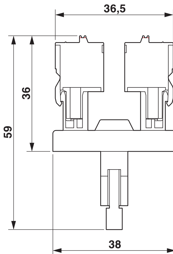
Dessin coté
