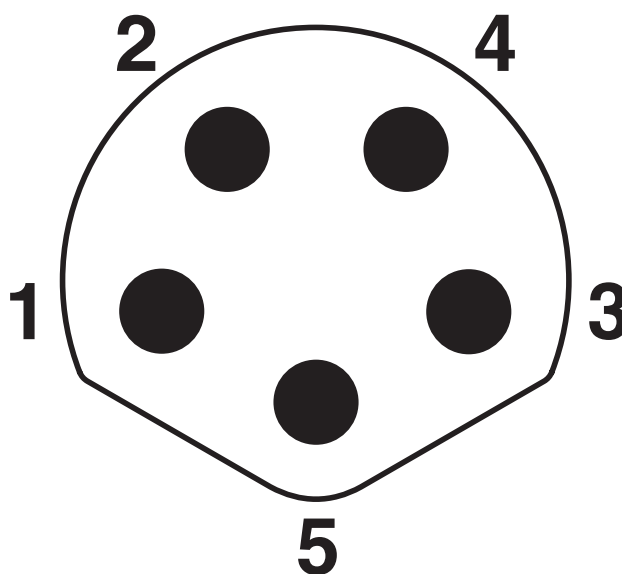
Esquema polos conector macho M8, 5 polos, codificado B, vista cara de machos
