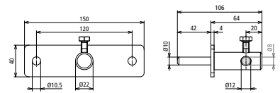
Maßbild ASK 8 150 40 2XB10.5 V2A
