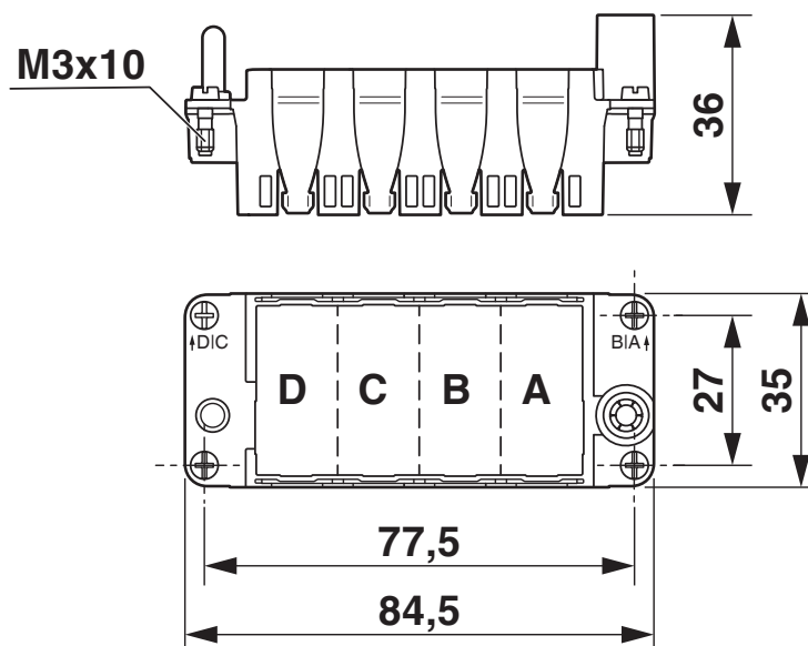
Dessin coté
