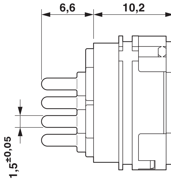
Dessin coté
