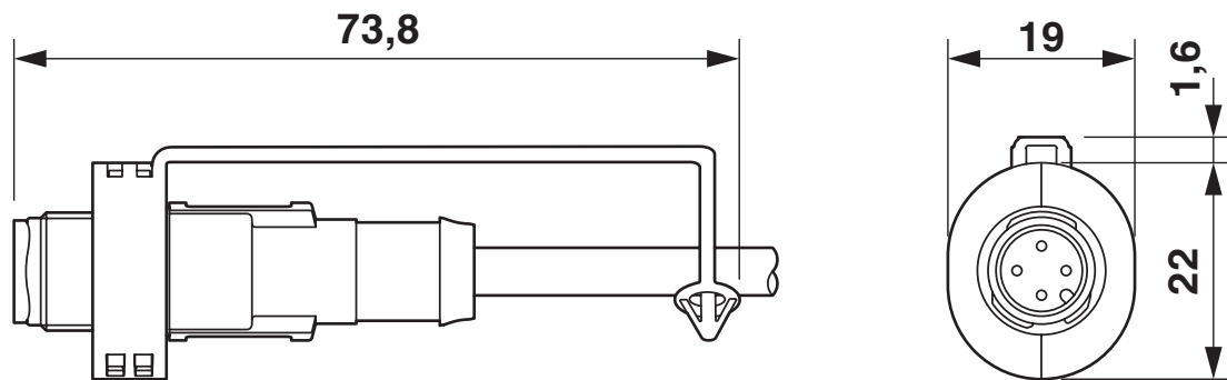
Maßzeichnung
