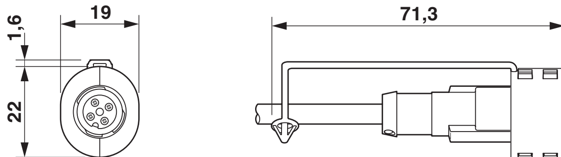
Maßzeichnung
