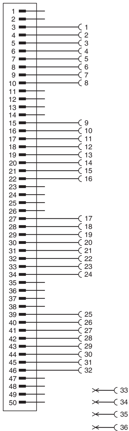
Diagrama eléctrico
