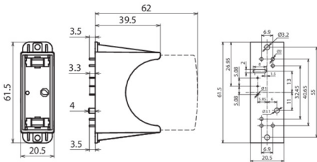
Dimensiones del DG PCB PV I 750 FM
