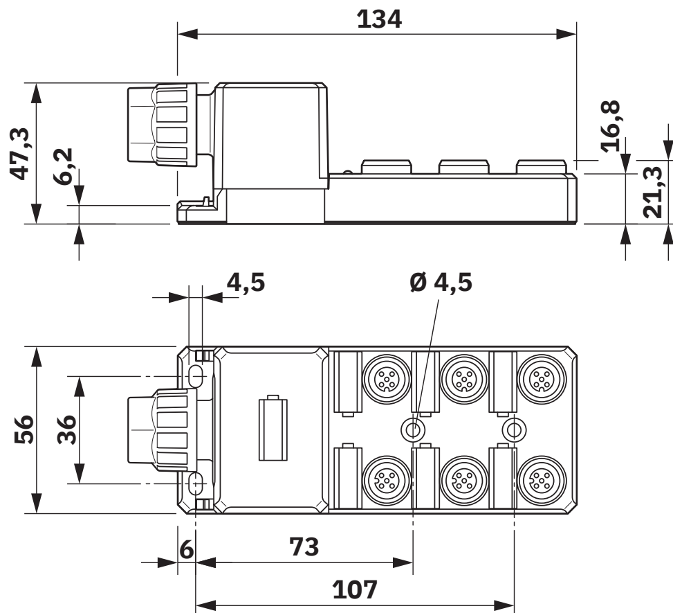
Dessin coté
