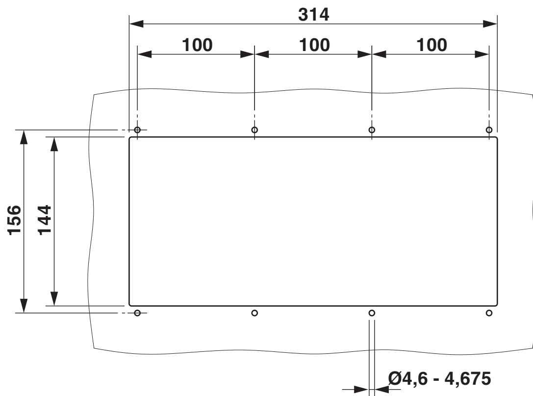
Plan de découpe de paroi
