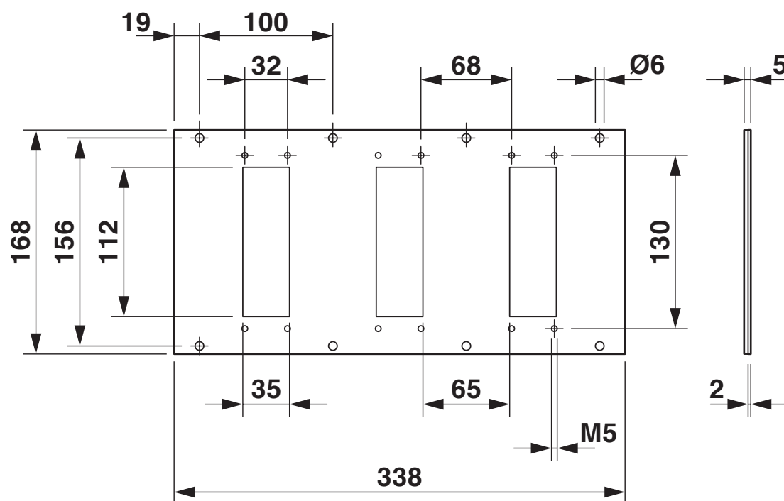
Dessin coté
