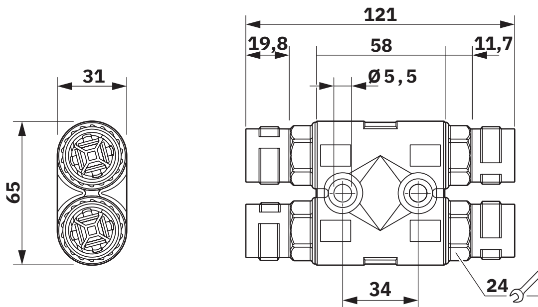
Maßzeichnung
