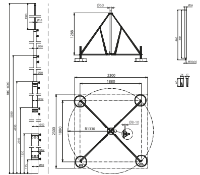
Maßbild FS T D50 1.8 8.0M AL VBS RA1330
