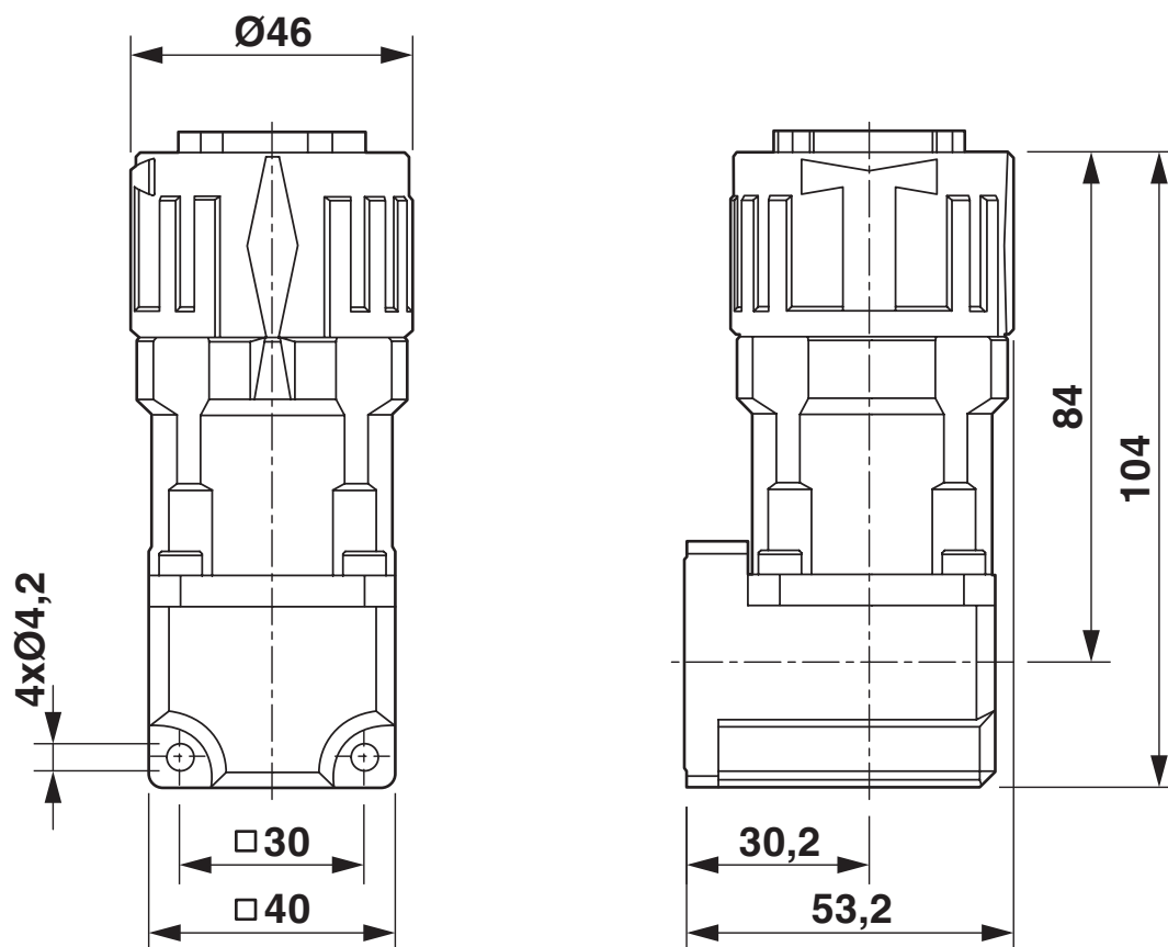
Dessin coté
