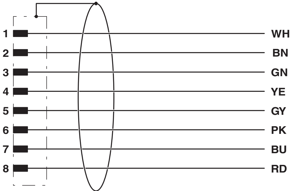
Kontaktbelegung des M12-Steckers
