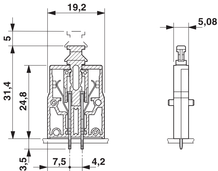
Maßzeichnung
