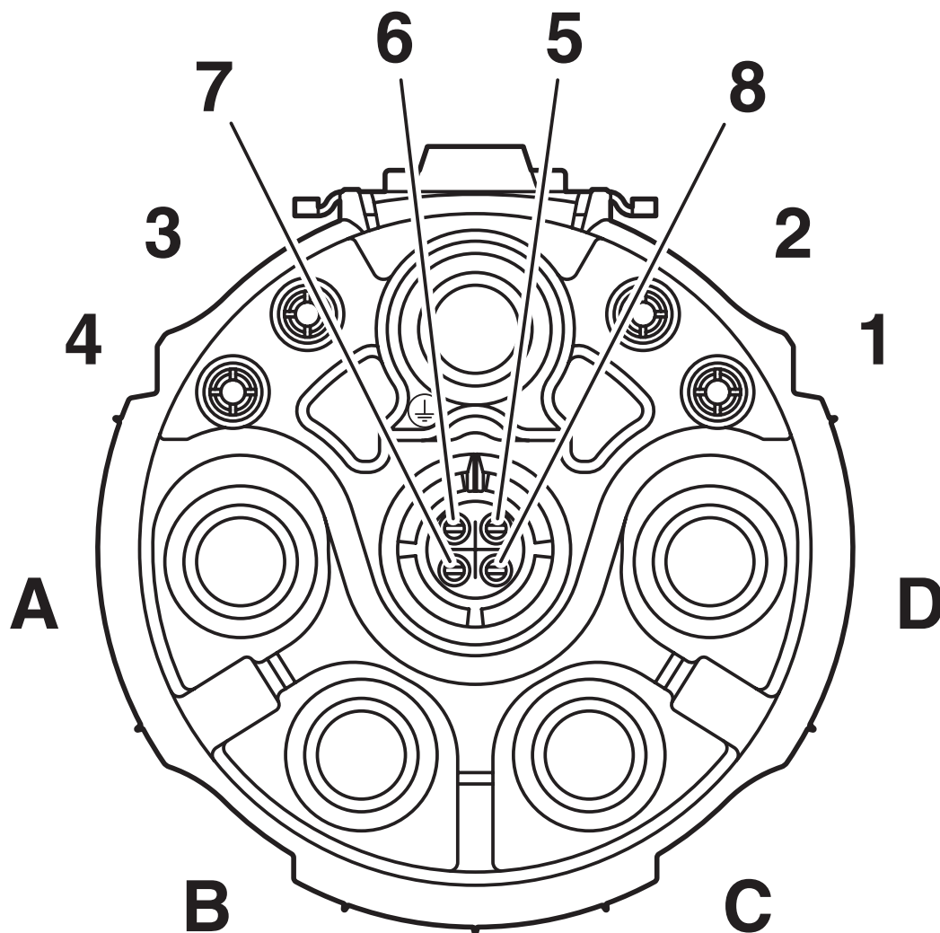
Schemazeichnung
