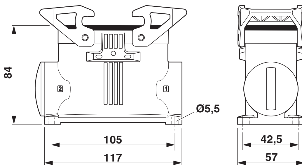
Dessin coté
