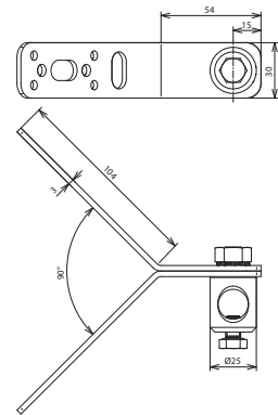
Maßbild EBW90 BB16 B5.1 6.5 11 V2A
