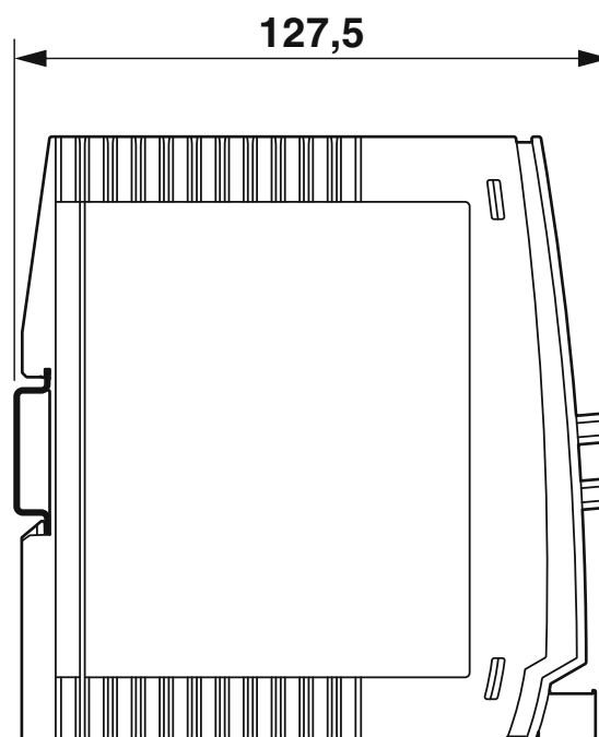
Dessin coté
