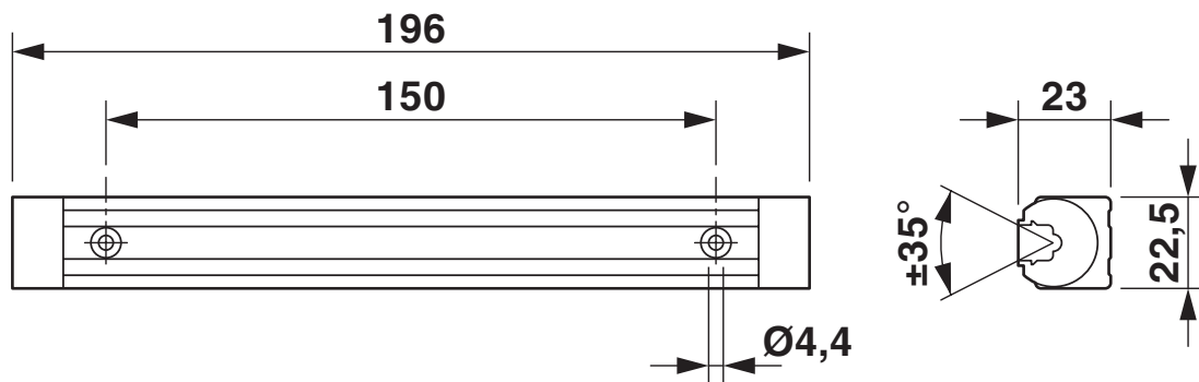
Maßzeichnung
