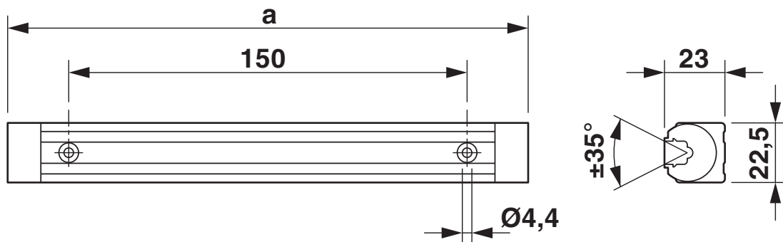
Maßzeichnung
