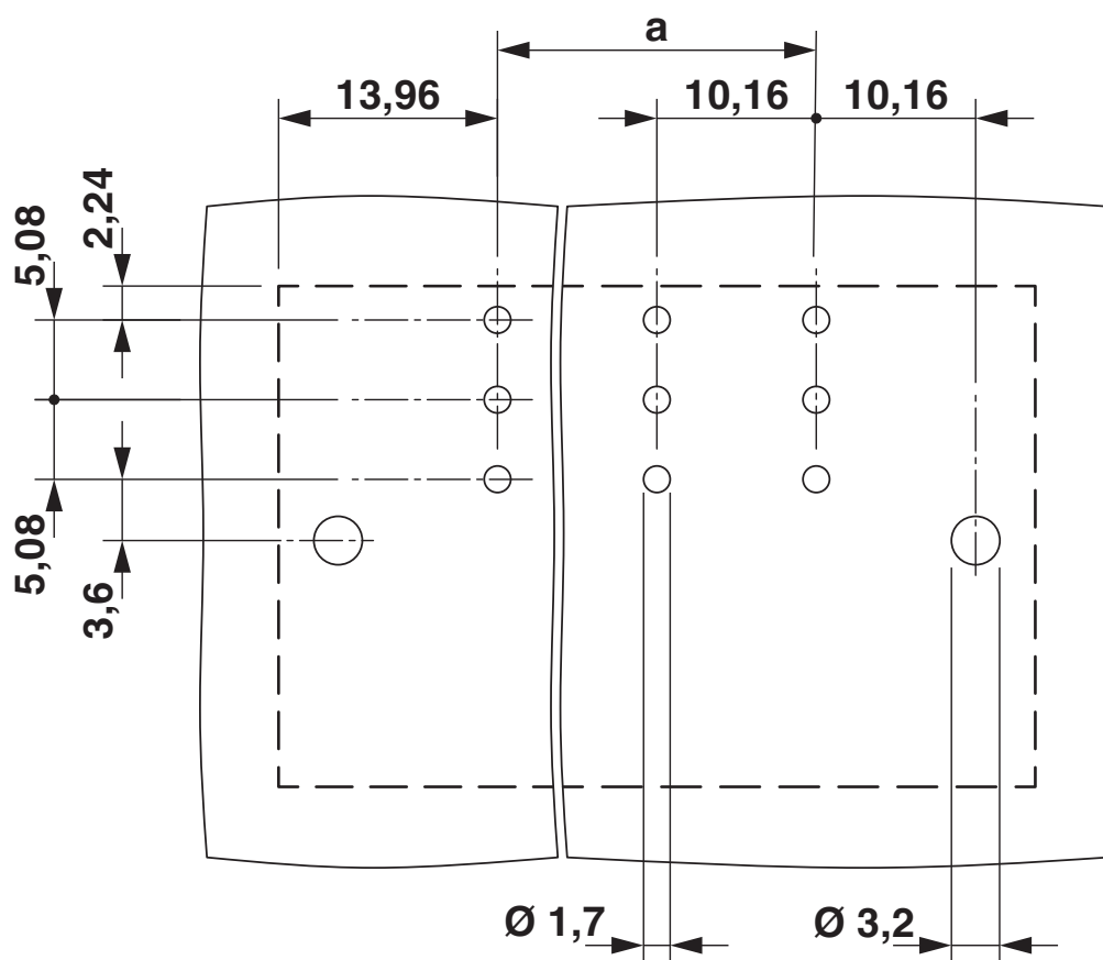
Esquema de taladros/geometría pads soldadura
