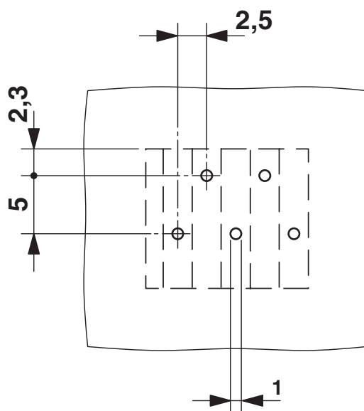
Bohrplan/Lötpadgeometrie
