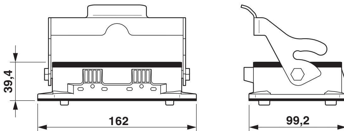
Maßzeichnung
