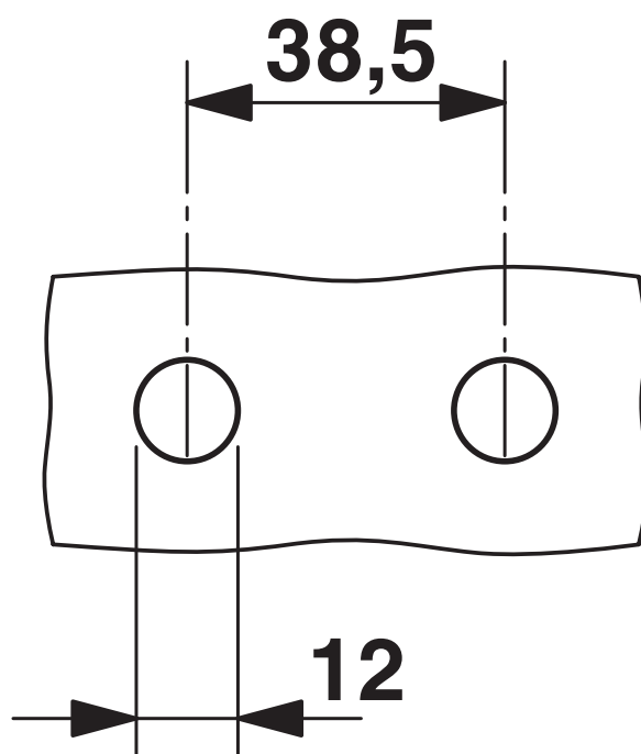
Dessin coté
